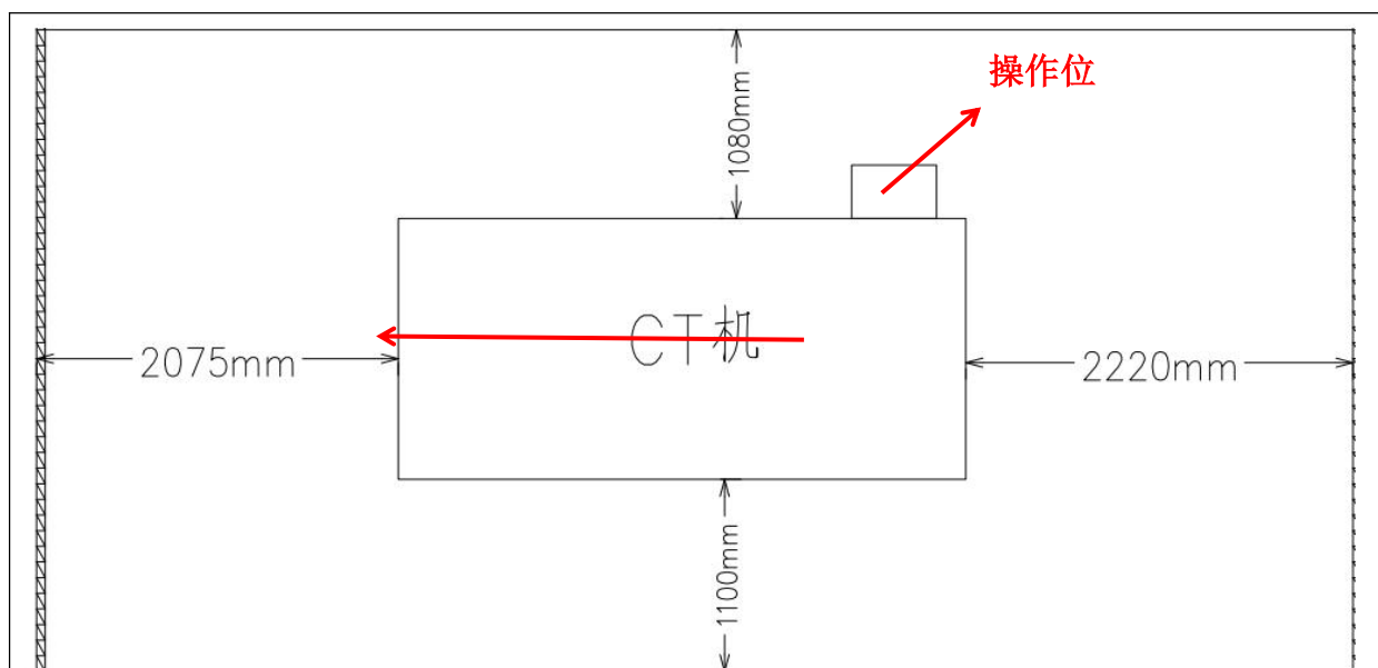
图 1-4 CT 检测区平面布置图
