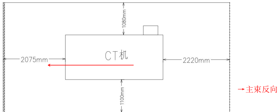
图 11-1 项目工业 CT 机的摆放位置图
