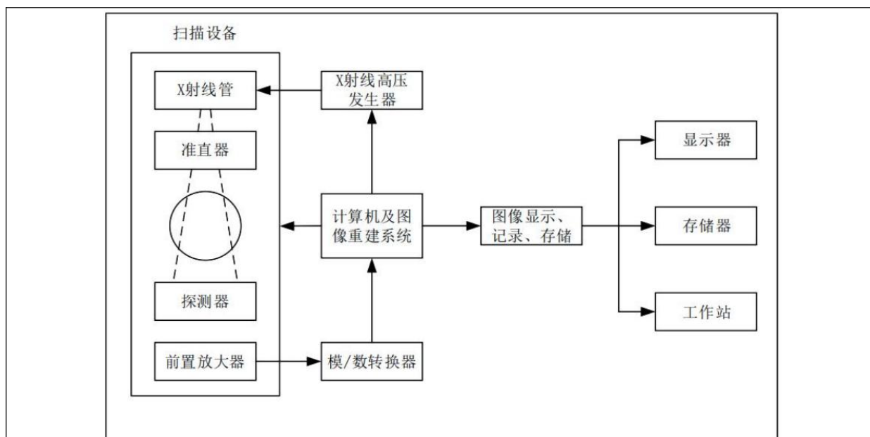
图 9-2 X 射线断层检查仪系统组成示意图
